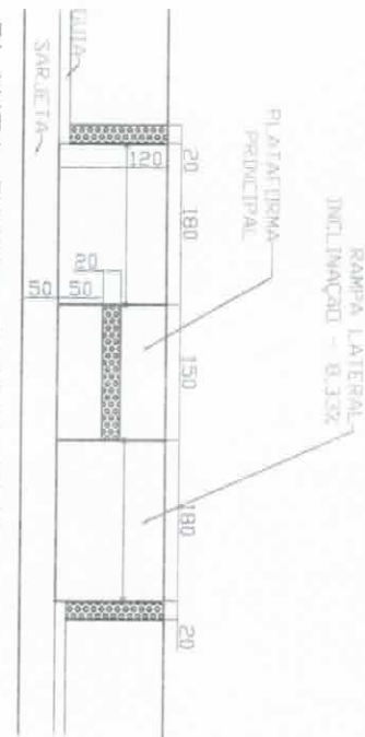
PLANTA BAIXA - DETALHE 2
